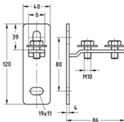
MPC-čelní příruba, příčná
