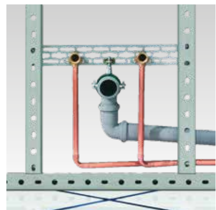
Předstěnová instalace: Předstěnová instalace s prvky StaboFix® v kombinaci s MPC-nosíky
